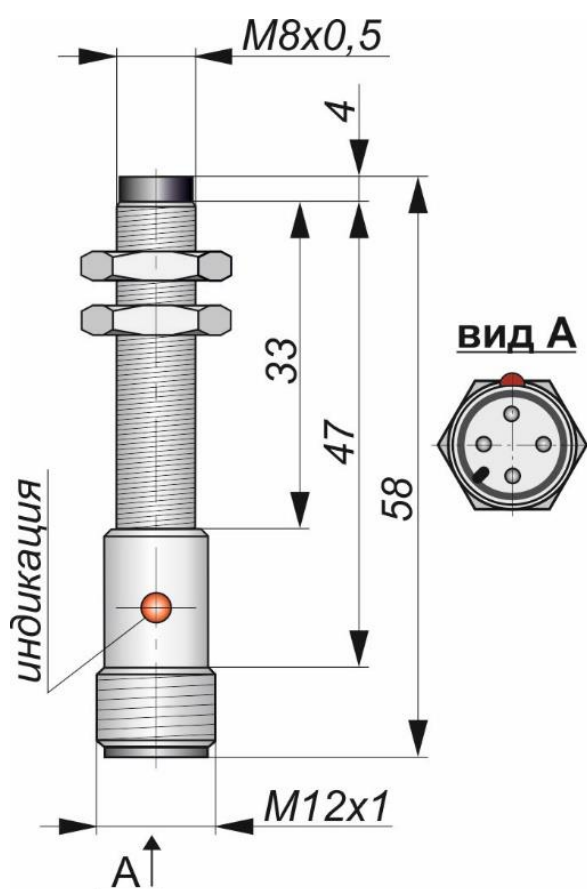
Габаритный чертеж
